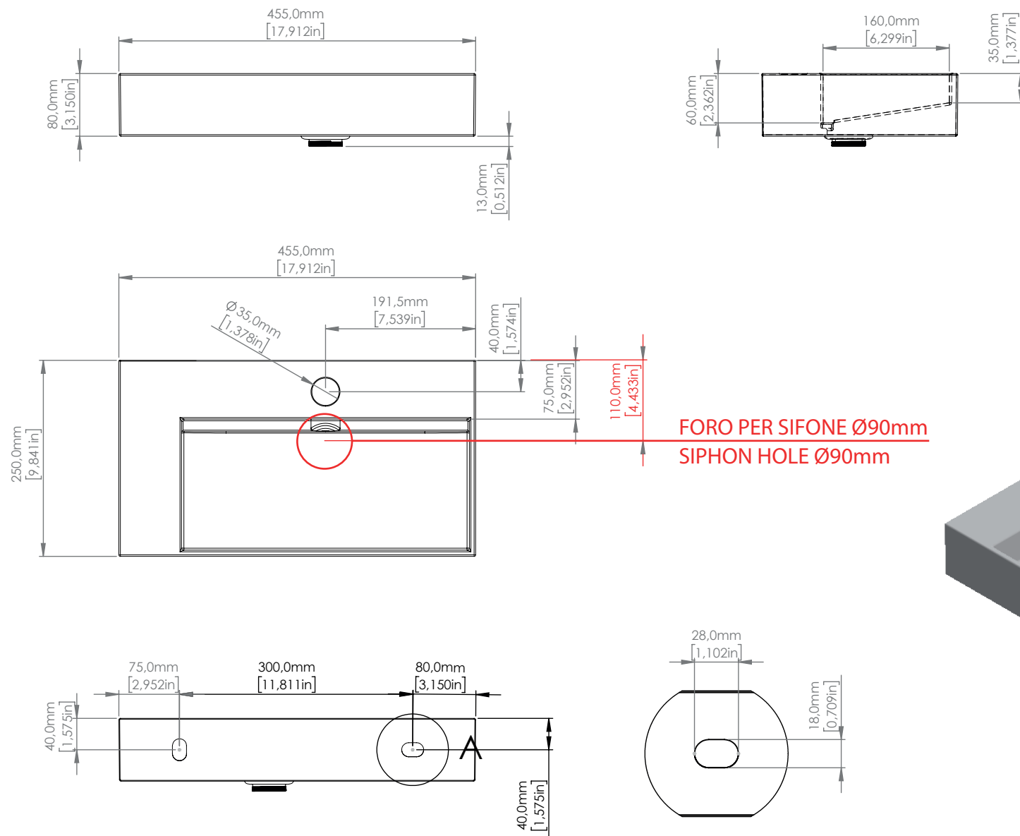
DETTAGLIO A SCALA 2 : 5
